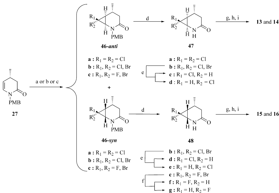
Scheme 8. Synthesis of 13–16 . Reagents: (a) \text{CHCl}_3 , 50% \text{NaOH} aq, aliquat-336 ( 46a-anti : 53%, 46a-syn : 14%); (b) \text{ClCHBr}_2 , 50% \text{NaOH} aq, \text{PhCH}_2\text{NET}_3\text{Cl} ( 46b-anti : 64%, 46b-syn : 18%); (c) \text{FCHBr}_2 , 50% \text{NaOH} aq, \text{PhCH}_2\text{NET}_3\text{Cl} ( 46c-syn : 15%); (d) \text{BF}_3\cdot\text{OEt}_2 , anisole, 100^\circ\text{C} (75–96%); (e) (\text{TMS})_3\text{SiH} , \text{BEt}_3 , toluene, room temperature ( 47c : 44%, 47d : 28%; 48d : 42%, 48e : 54%); (f) \text{Ph}_3\text{SnH} , \text{AIBN} , benzene, 80^\circ\text{C} ( 48g : 22%); (g) \text{Et}_3\text{O}^+\text{BF}_4^- , \text{CH}_2\text{Cl}_2 ; (h) \text{NH}_3 , \text{EtOH} ; (i) 4 M \text{HCl} dioxane (9–48% in three steps).
